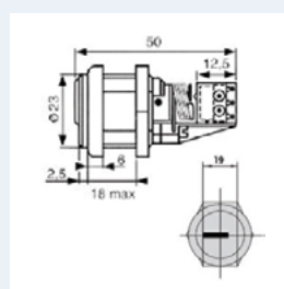
Contacteur
