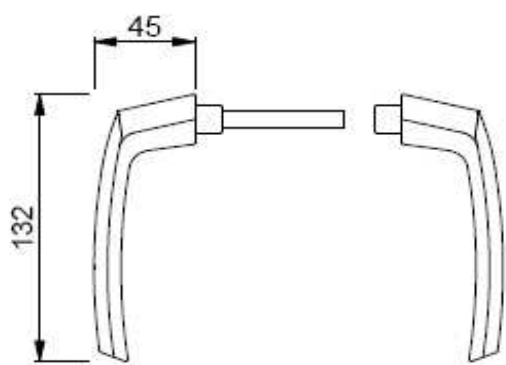
Béquille sur rosace
