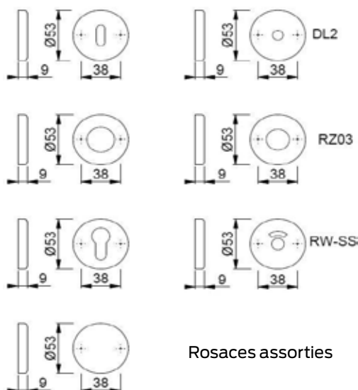
Version béquille/béquille - Condamnation
