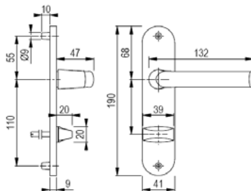
Version béquille/béquille - Condamnation
