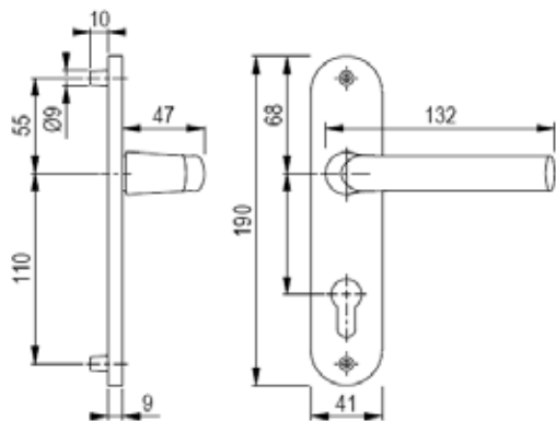
Version béquille/béquille - Clé I
