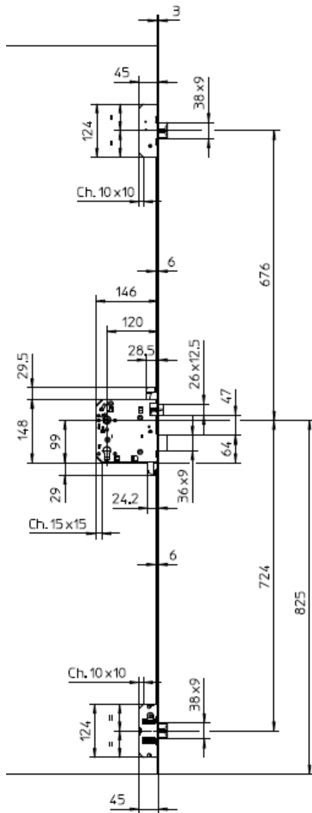
Serrure 3 coffres avec 3 pènes rectangulaires Longueur 1700mm
