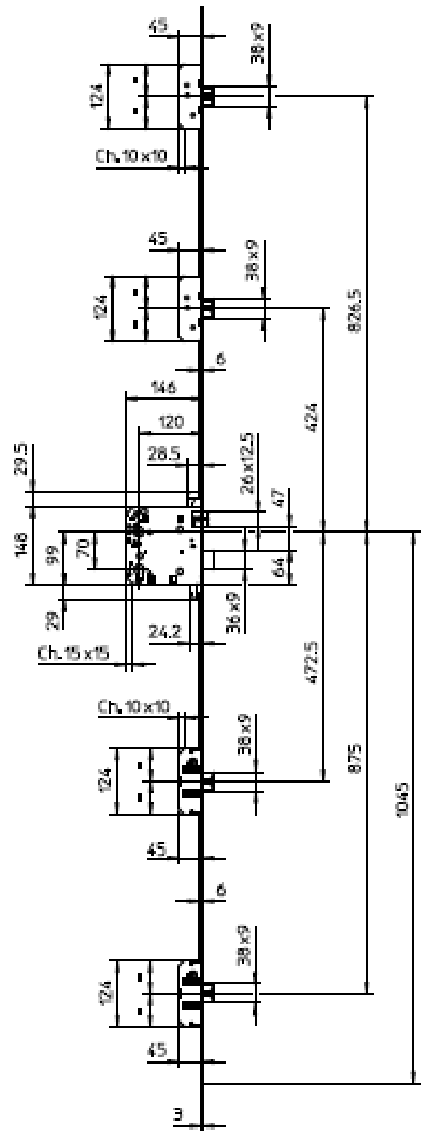
Serrure 5 coffres avec 5 pènes rectangulaires Longueur 2400mm
